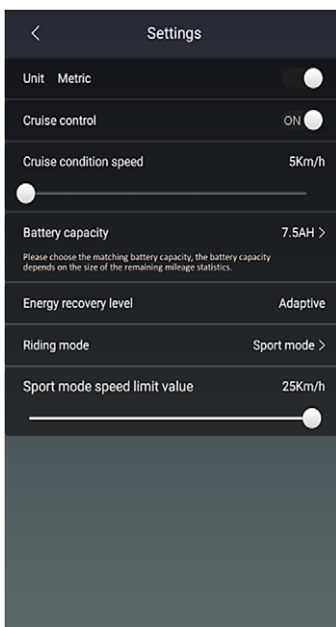
Stránka nastavení
